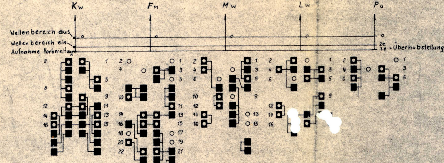
Schalter in Überhub Stellung gezeichnet
